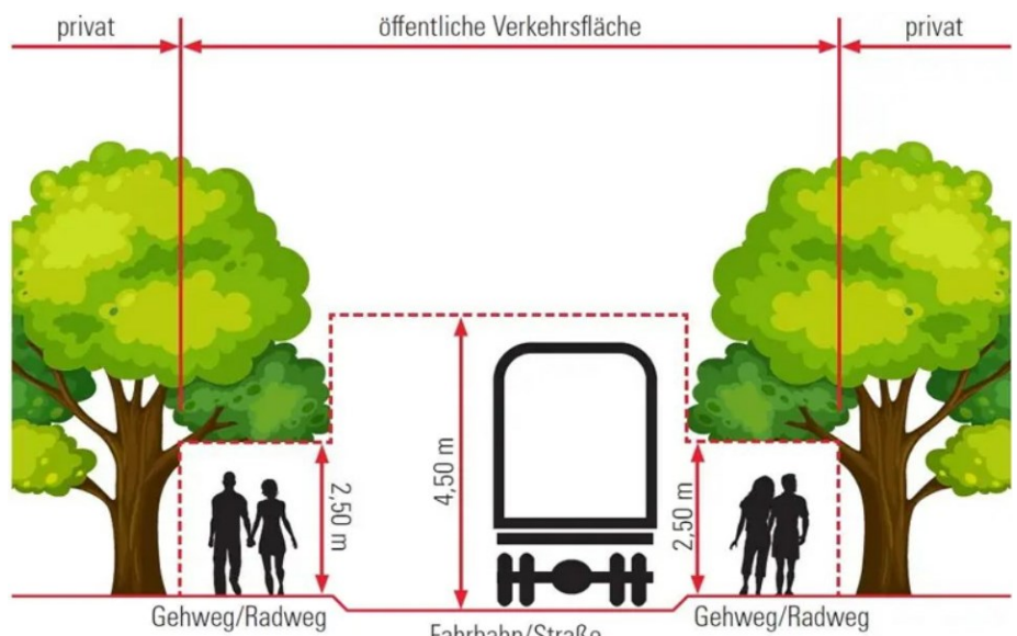
Lichttraumprofil
